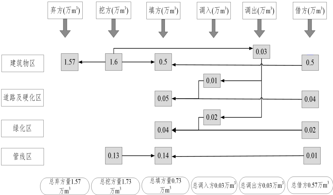
图 2.4-1 土方流向框图
