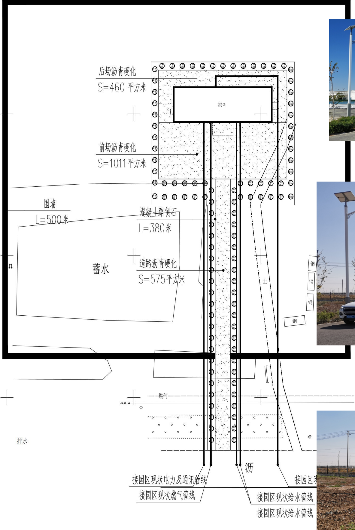
附图 2 水土流失防治责任范围及水土保持措施布设竣工验收图
