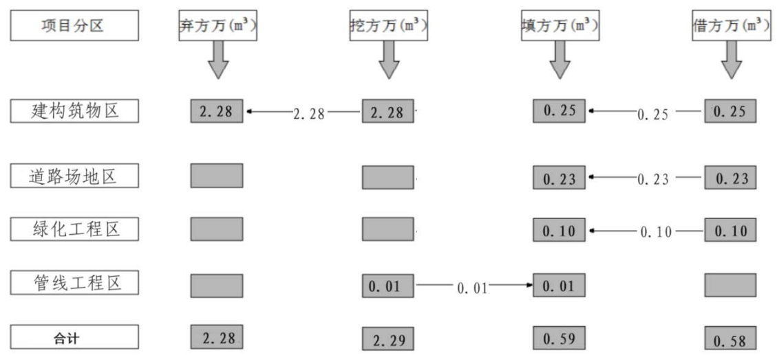
图 2-9 工程土方流向框图
