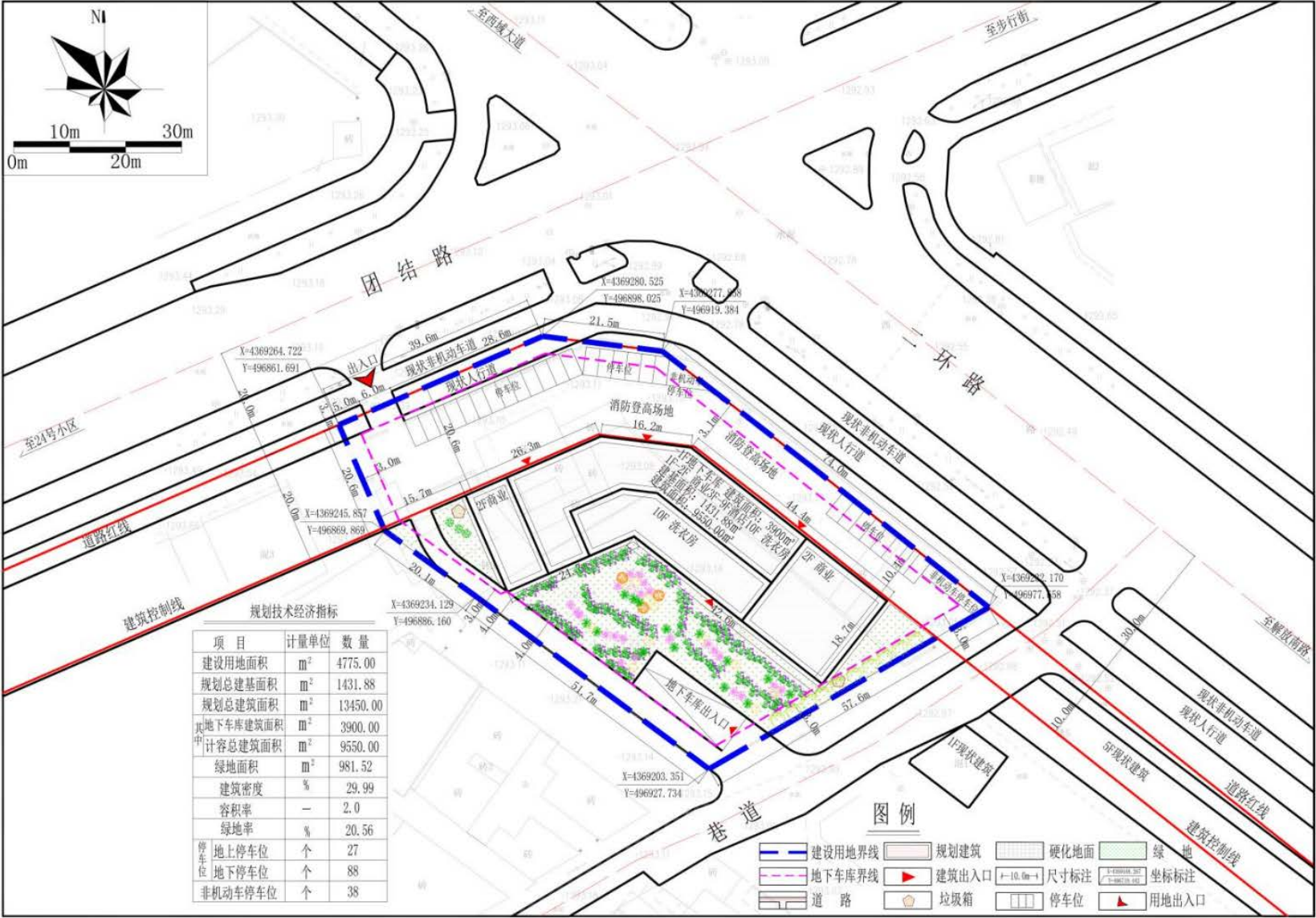
图 2-3 项目平面布置图
