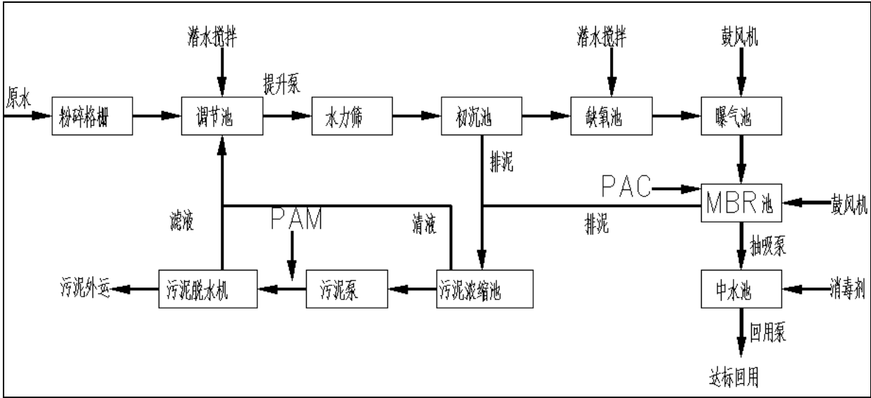
图 2-8 污水处理及中水回用系统工艺流程
