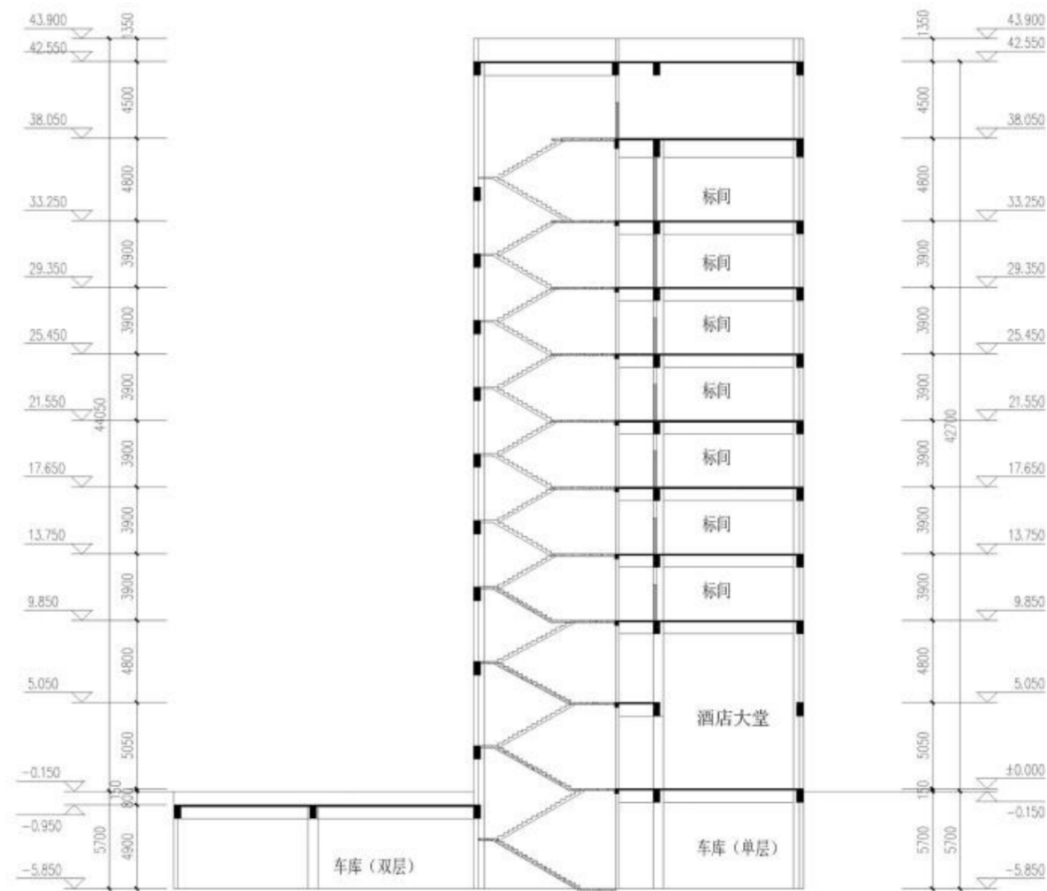
图 2-4 商业楼立面图 1: 100
