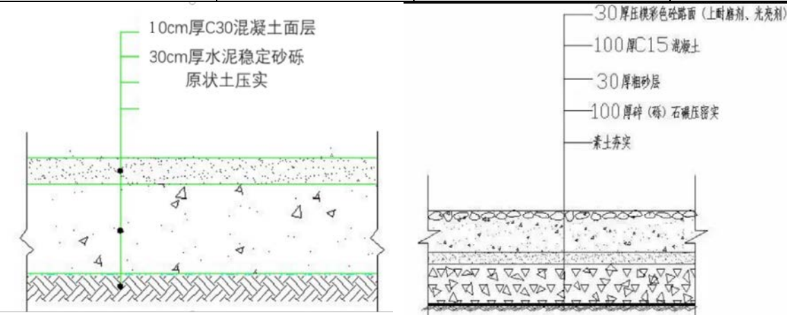
图 2-6 路面混凝土结构做法
