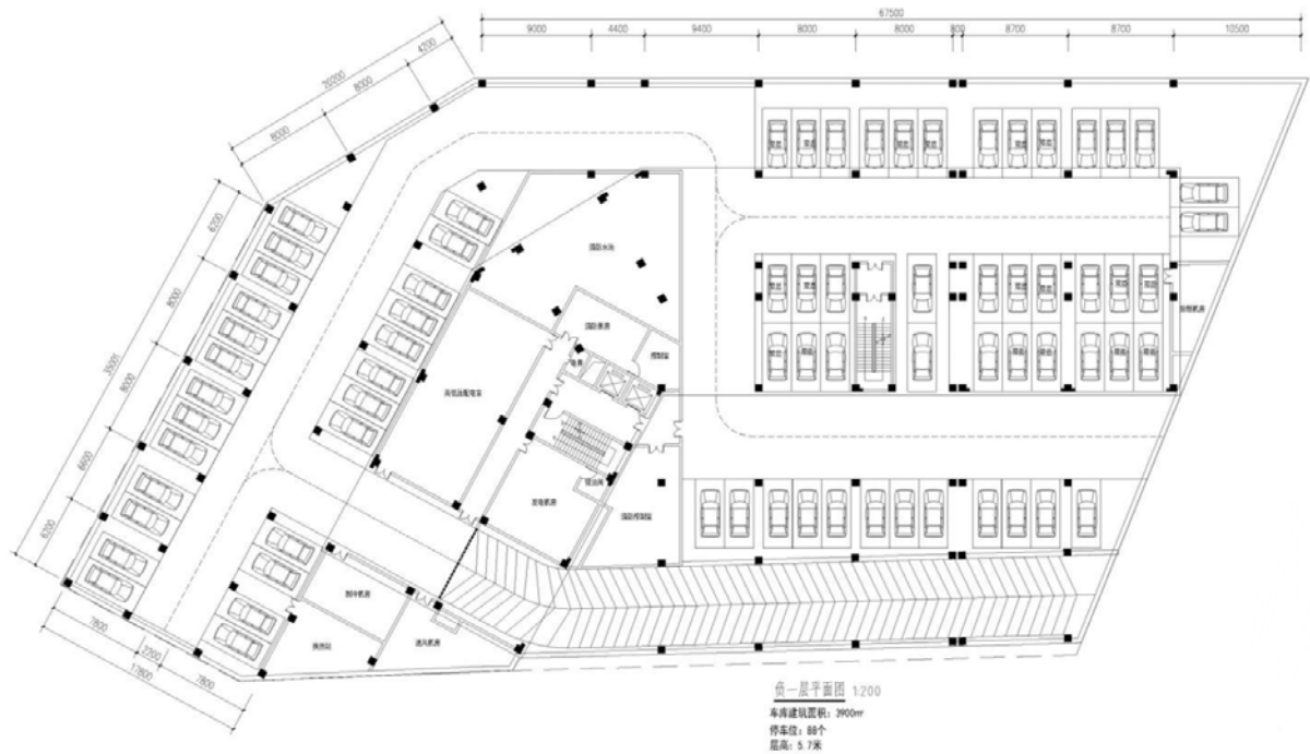
图 2-5 一楼平面图 1: 100
